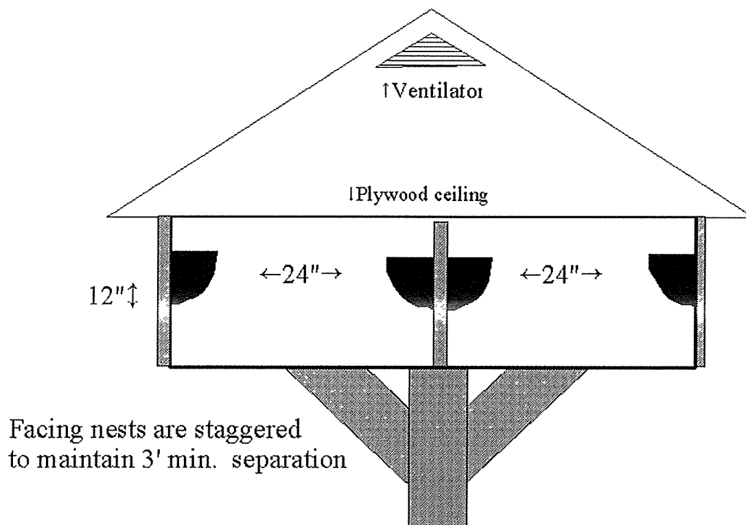
Figuur 22. Schematische voorstelling van houten afdak met daaronder kunstnesten voor Boerenwaluw, bevestigd aan houten dwarsplanken (Bron: www.americanartifcats.com )
