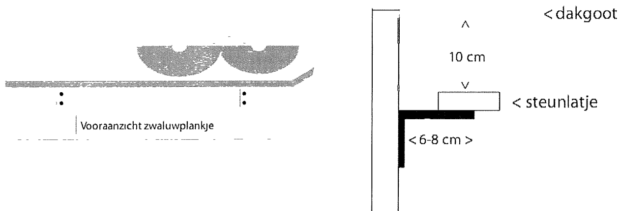
Figuur 15 Schets vooraanzicht en zijaanzicht van een steunlatje onder nesten van Huiszwaluw (Anoniem, 2010)
